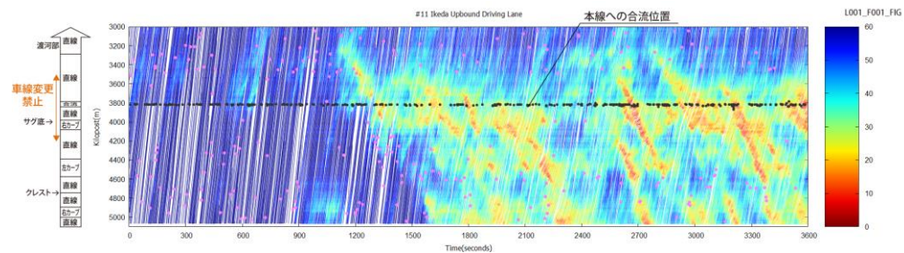
速度のタイムスペース図
