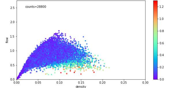
密度と流率の分布
